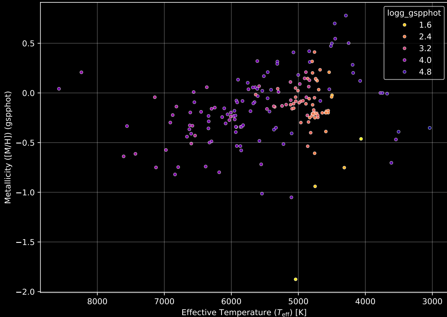
APOGEE DR17 Field: [CVZTILE_093+27_btx] Stellar Population Parameters (n= 181)
